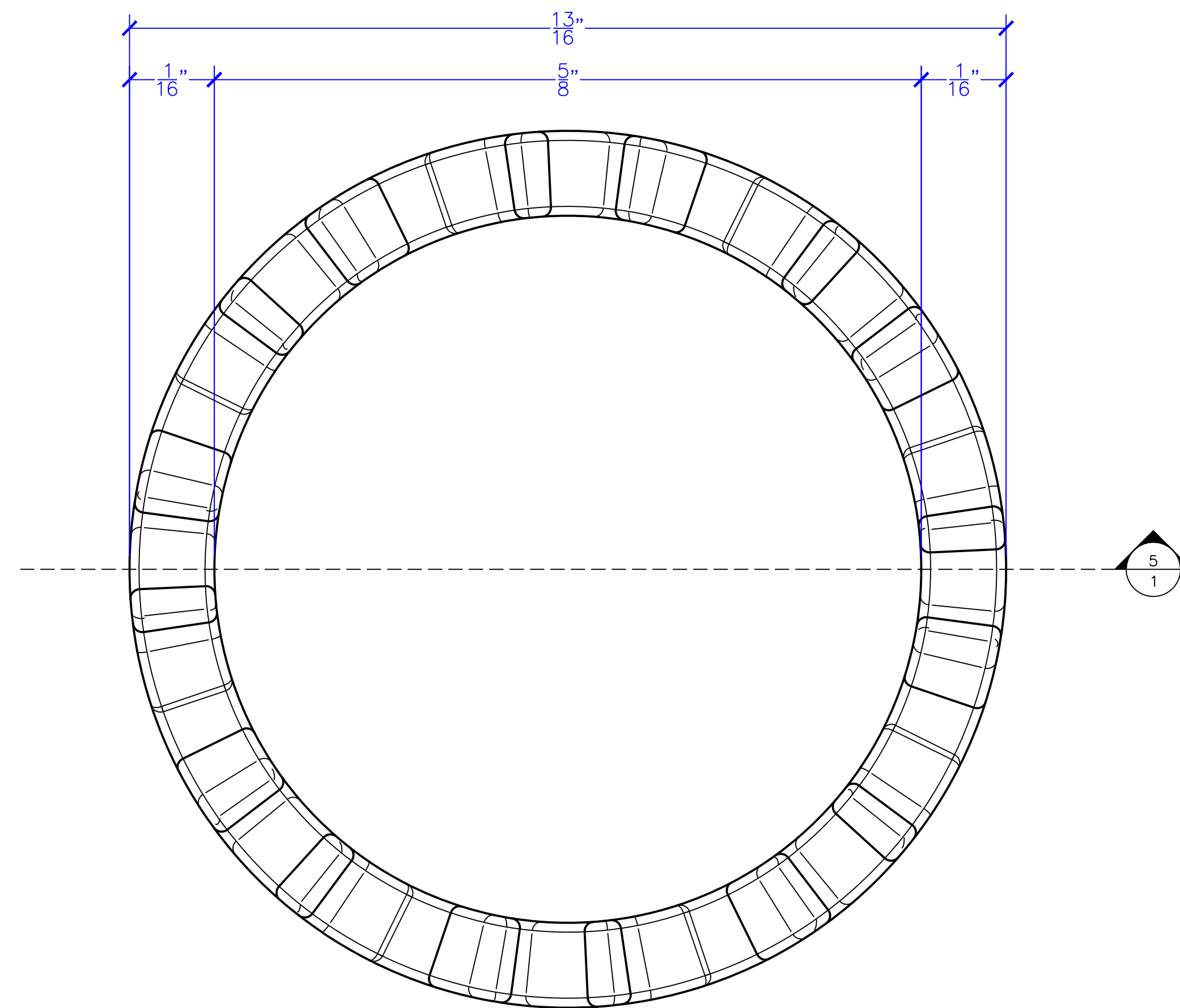
3 TOP VIEW Scale: 10:1
