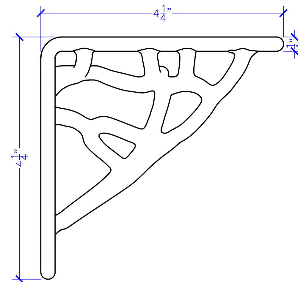
4 LEFT VIEW Scale: 1" = 1"
